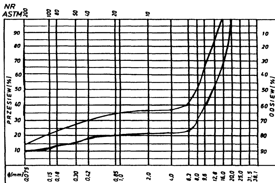
Krzywe graniczne uziarnienia mieszanki mineralnej 0+20 mm o nieciągłym uziarnieniu do warstwy ścieralnej z betonu asfaltowego dla KR 3-6
