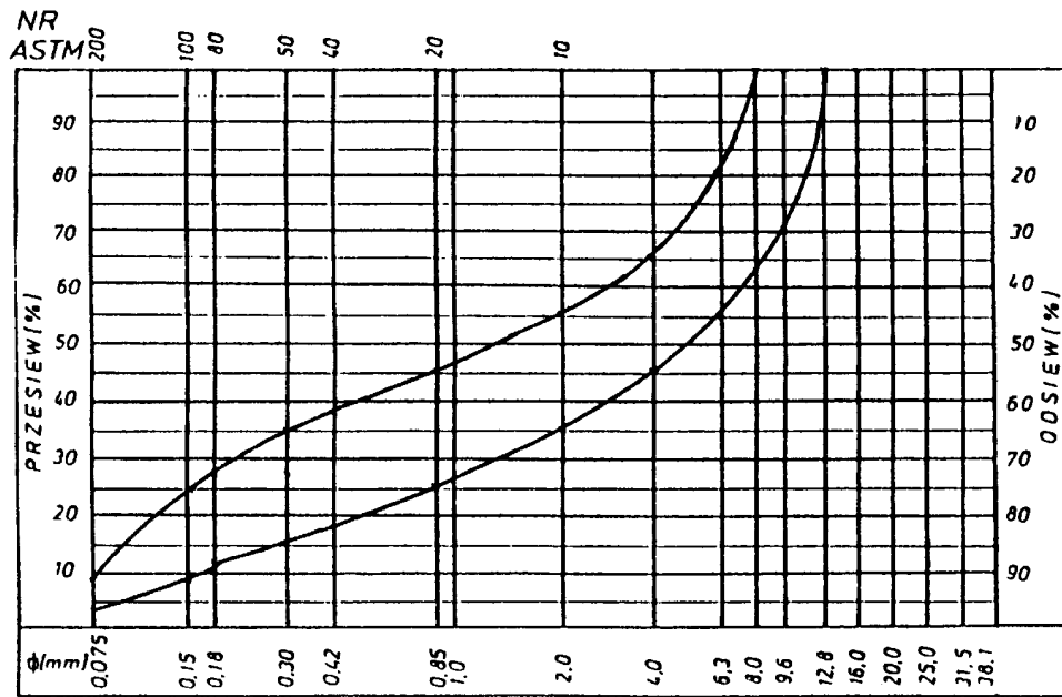
Krzywe graniczne uziarnienia mieszanki mineralnej 0+12,8 mm do warstwy wiążącej, wyrównawczej i wzmacniającej z betonu asfaltowego dla KR 1-2
