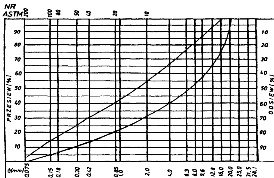
Krzywe graniczne uziarnienia mieszanki mineralnej 0+20 mm do warstwy wiążącej, wyrównawczej i wzmacniającej z betonu asfaltowego dla KR 1-2
