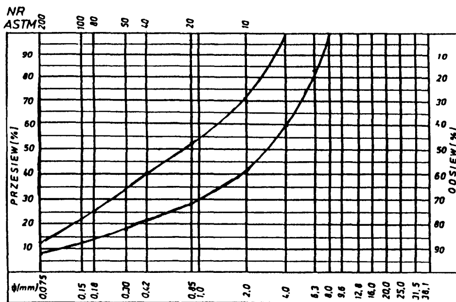
Krzywe graniczne uziarnienia mieszanki mineralnej 0+8, 0+6,3 mm do warstwy ścieralnej z betonu asfaltowego dla KR 1-2
